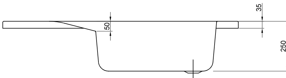
Presjek A-A
