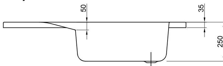
Presjek A-A
